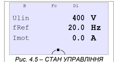
Рис. 4.5 – СТАН УПРАВЛІННЯ
