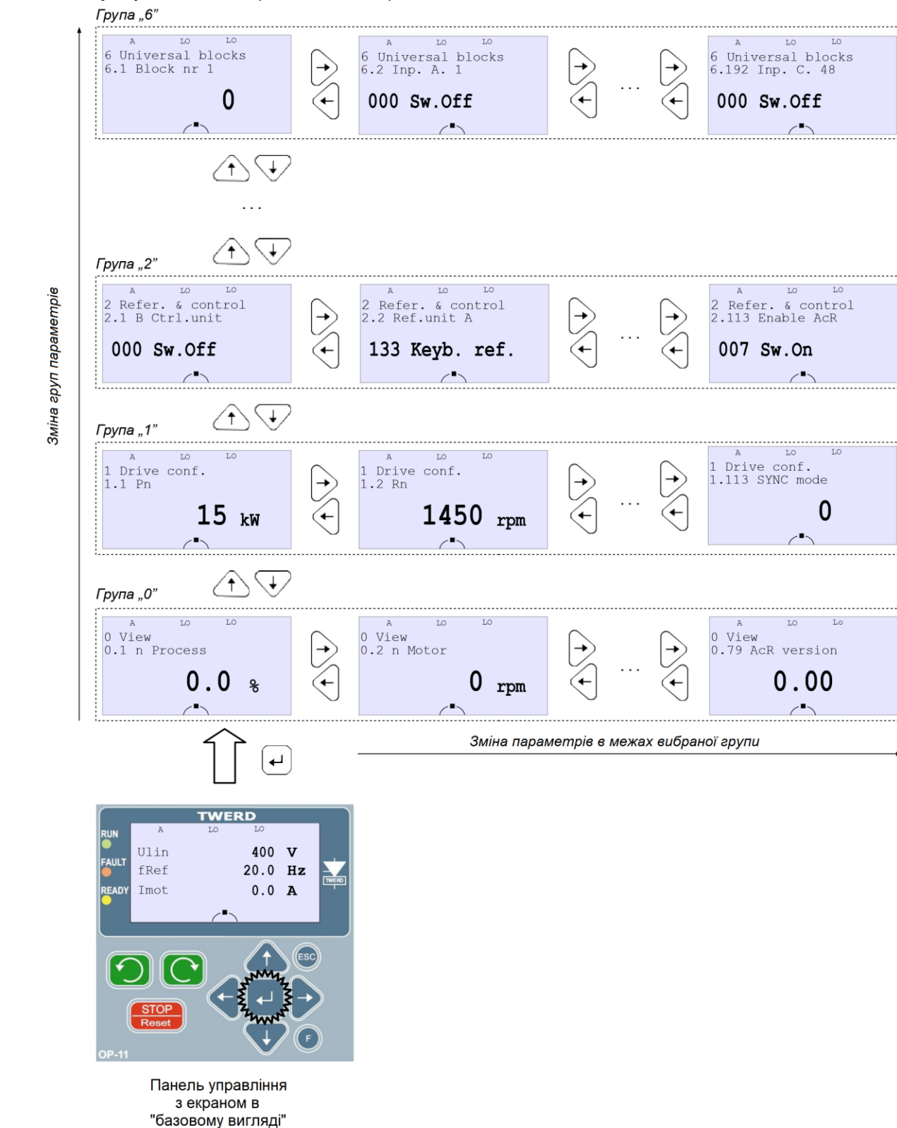
Рис. 3.3 - Схема обслуговування панелі управління ОП-11
