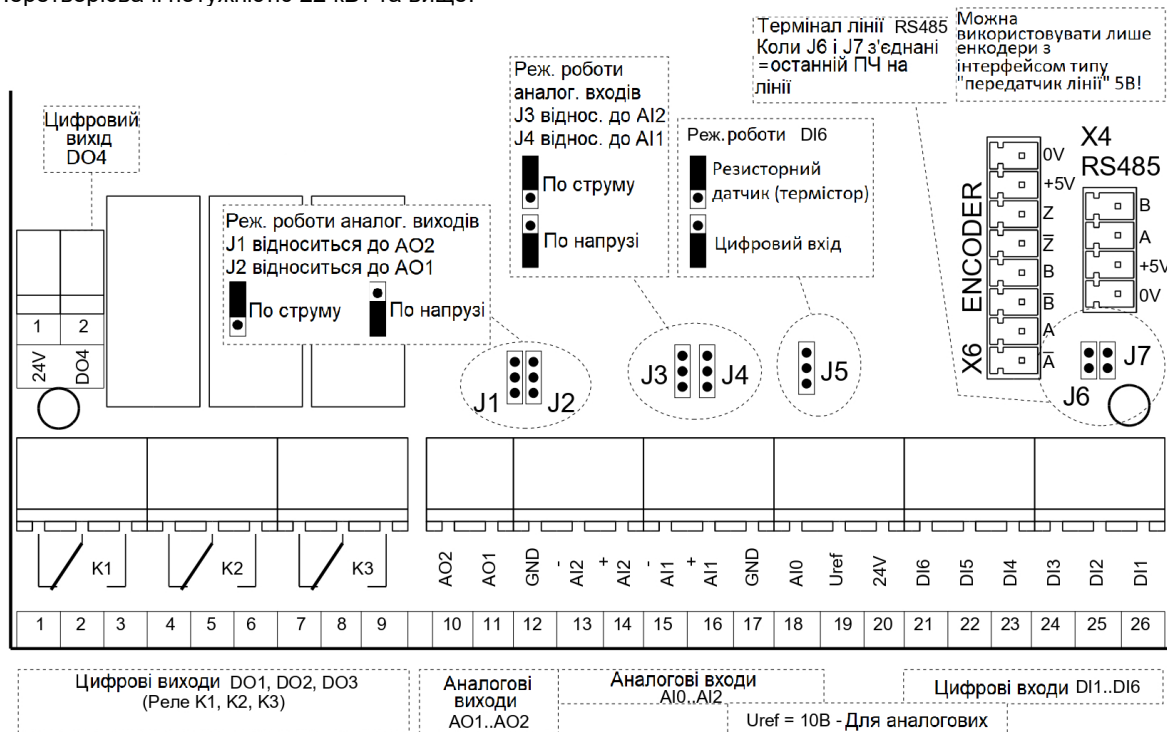
Рис. 2.6б – Клемники системи управління перетворювача MFC710 та перемикачі конфігурації. Роз'єм енкодера та RS485. Варіант для потужності 22 кВт та вище.
