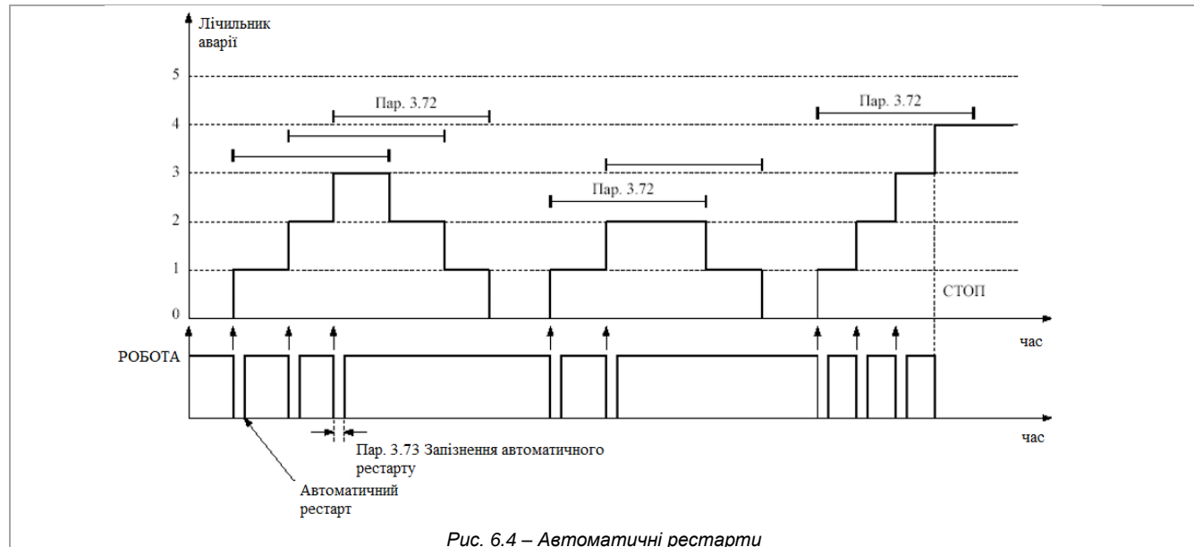
Рис. 6.4 – Автоматичні рестарти
