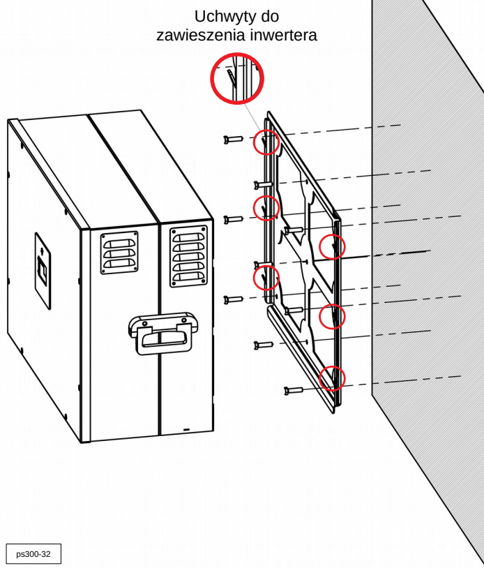
Rys.4.11. Montaż inwertera na ścianie – moce 12 kW - 30 kW
