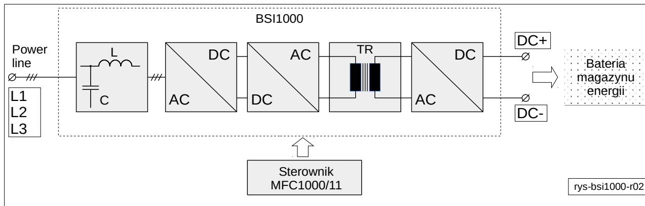
Rys. 2.1. Schemat blokowy BSI1000
