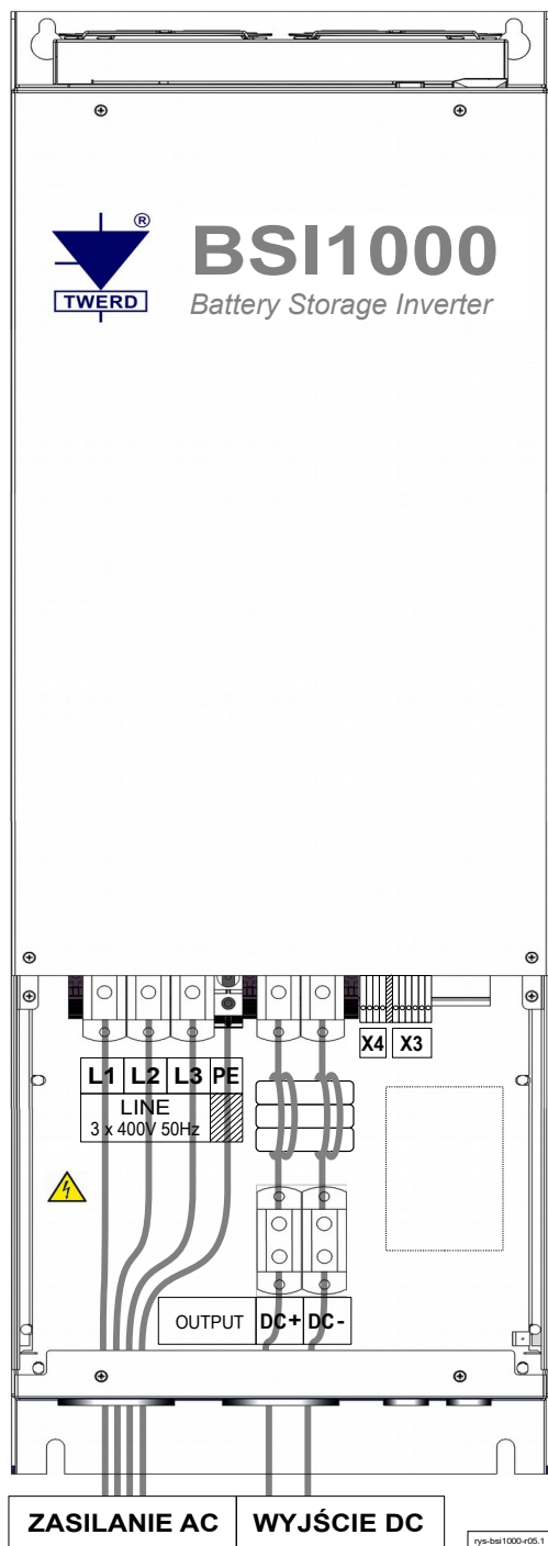
Rys. 5.1. Zaciski przyłączeniowe obwodu mocy
