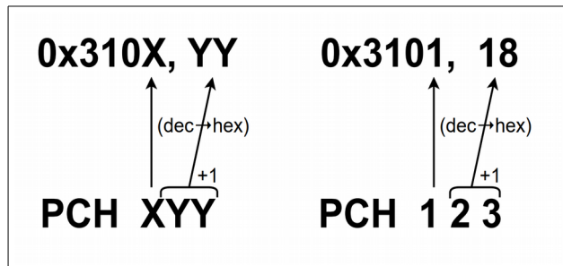
Rys 8. Adresowanie PCH
