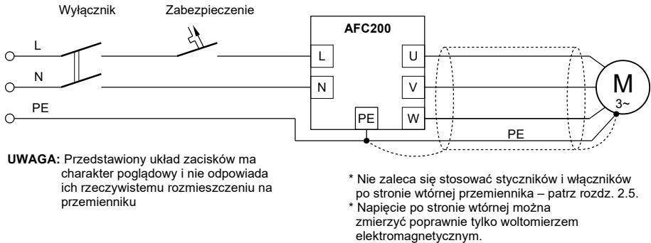
Rys. 2.3. Podłączenie obwodów silnopiędowych do przemiennika AFC200
