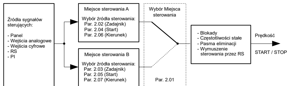
Rys. 5.1. Uproszczona struktura sterowania układu AFC200
