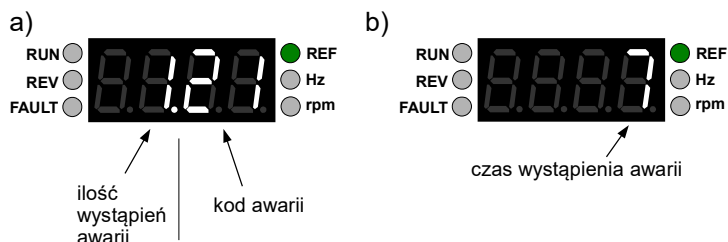
Rys. 8.1. Przykładowa awaria odczytana z par. 3.80 (rys. a) wraz z czasem wystąpienia odczytanym z par. 3.81 (rys. b)
