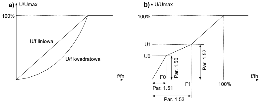
Rys. 5.3. Charakterystyka liniowa i kwadratowa (a), kształtowanie charakterystyki U/f (b)
