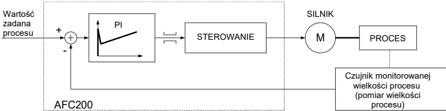
Rys. 6.1. Wykorzystanie regulatora PI do regulacji monitorowanej wielkości procesu
