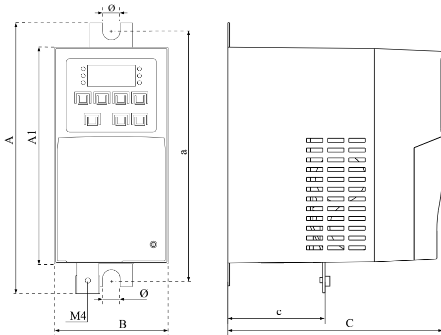
Rys. 2.2. Wymiary przemienników AFC200
