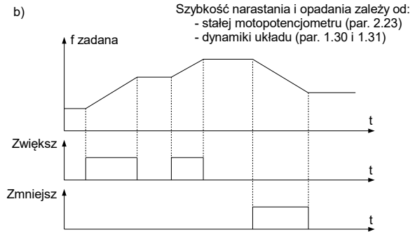
Rys. 5.5. a) - podłączenia na listwie zaciskowej X1, b) - ilustracja działania układu motopotencjometr
