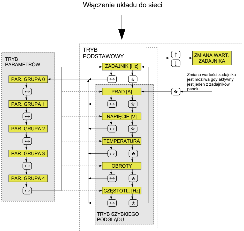
Rys. 3.2. Schemat obsługi panelu sterującego
