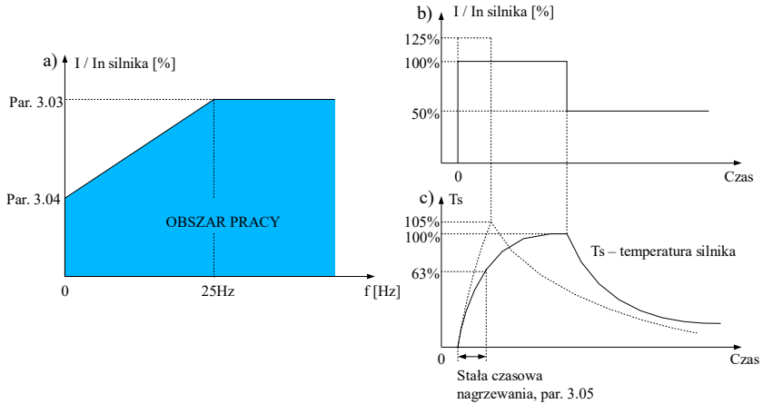
Rys. 5.7. Definiowanie obszaru pracy długotrwałej (a), zależność obliczonej temperatury silnika od prądu (b) i (c)
